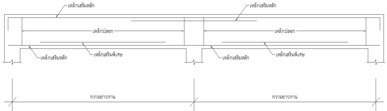
รูปที่ 3.3 แสดงการเสริมเหล็กคาน
