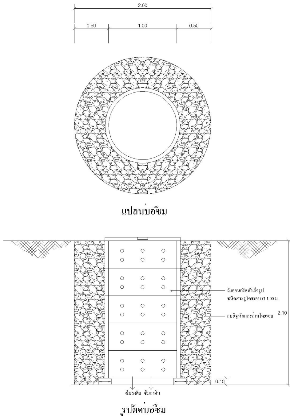
รูปที่ 2.7 รูปแปลนและรูปตัดบ่อซึม ที่มา : วิเชียร ปัญญาจักร
