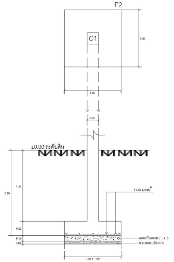
แบบขยายฐานราก F2
