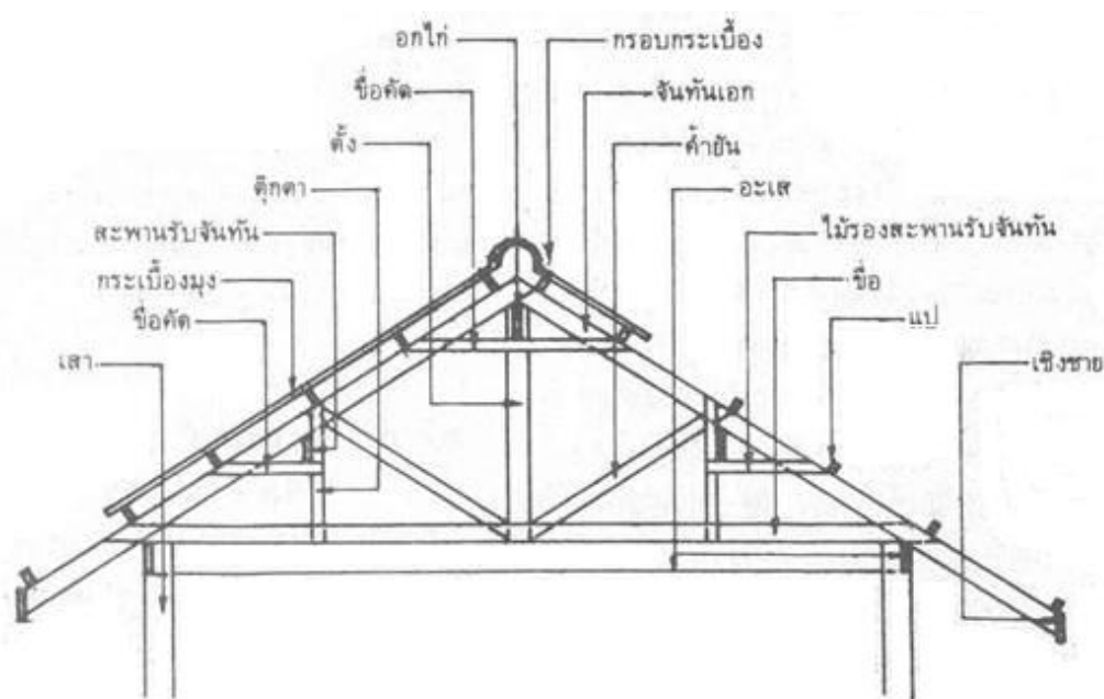
รูปที่ 3.11 แสดงรูปตัดด้านหน้าของโครงสร้างหลังคา
