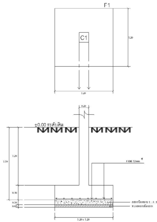
แบบขยายฐานราก F1
