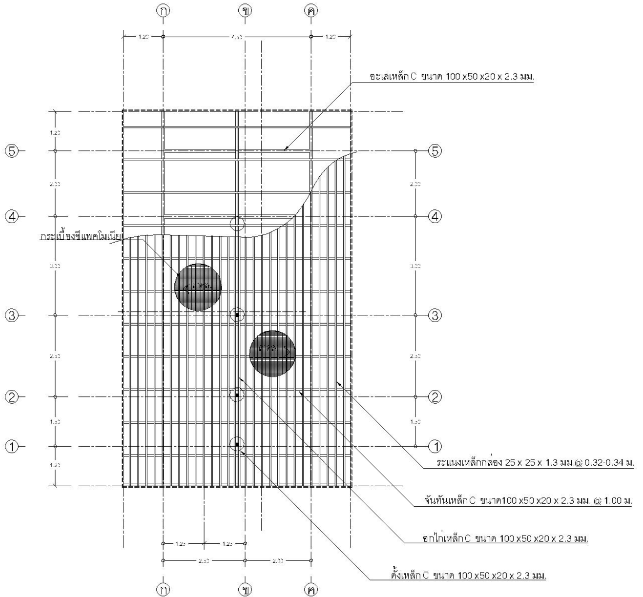
ผังโครงสร้างหลังคา มาตราส่วน 1 : 100
