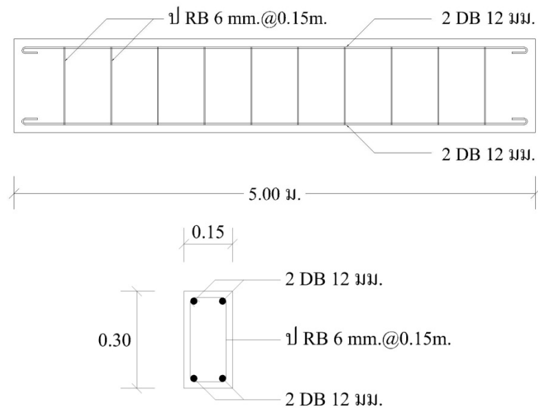
รูปที่ 3.4 แสดงรูปตัดคานตามความยาวและรูปตัดตามขวาง
