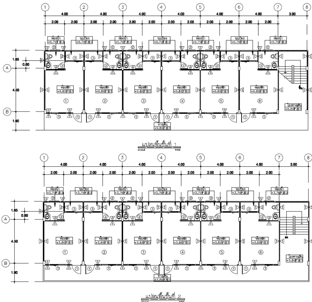
รูปที่ 1.3 แปลนพื้นที่ 1 และ แปลนพื้นที่ 2 ของอาคารหอพัก คสล. 2 ชั้น 6 หน่วย
