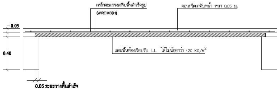
รูปที่ 3.10 แสดงแปลนโครงสร้างพื้นสำเร็จรูปและแบบรูปตัดพื้นสำเร็จ ที่มา : วิเชียร ปัญญาจักร
