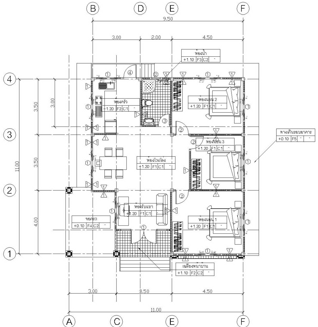
รูปที่ 4.4 แสดงแปลนพื้นชั้นล่าง
