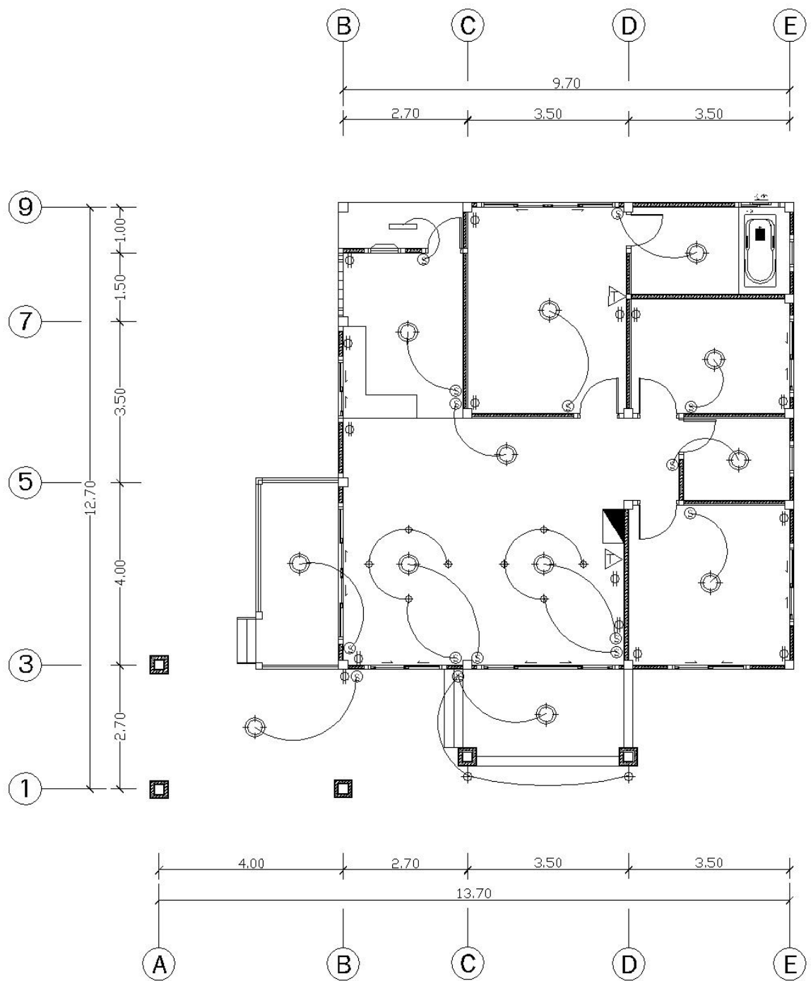
แบบแสดงแปลนไฟฟ้า มาตราส่วน 1 : 100
