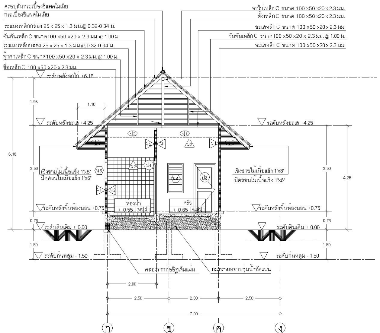
รูปตัด แนว A-A
