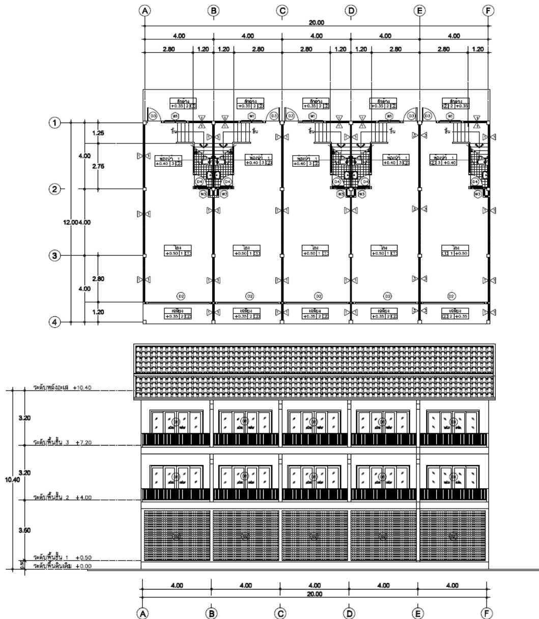
รูปที่ 1.2 แปลนพื้นที่และรูปด้านของอาคารพาณิชย์ 3 ชั้น 5 คูหา
